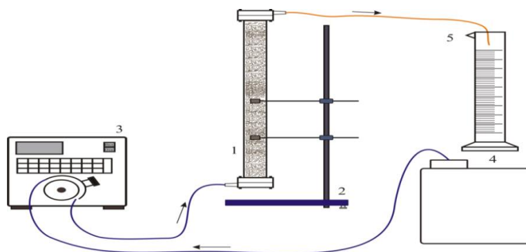
1 – сорбционная колонка; 2 – штатив; 3 – перистальтический насос; 4 – буферная емкость; 5 – мерный цилиндр для сбора маточников.
