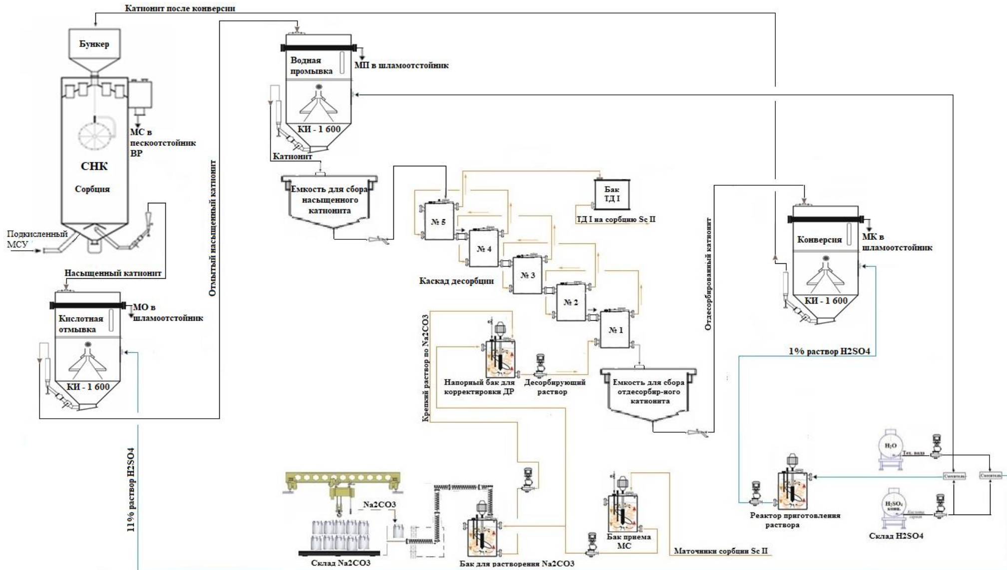
Рисунок 54– Принципиальная аппаратная схема технологии извлечения скандия (I этап концентрирования) из маточников сорбции урана
