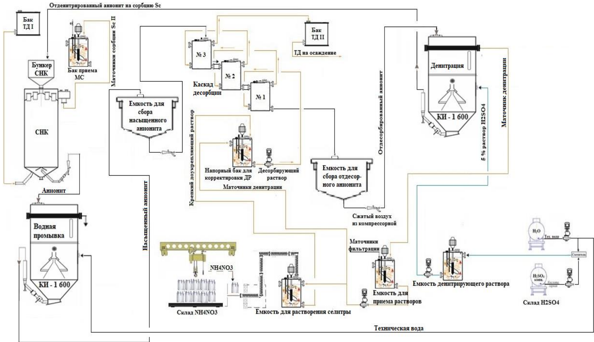
Рисунок 55 – Принципиальная аппаратная схема технологии извлечения скандия (II этап концентрирования) из маточников сорбции урана
