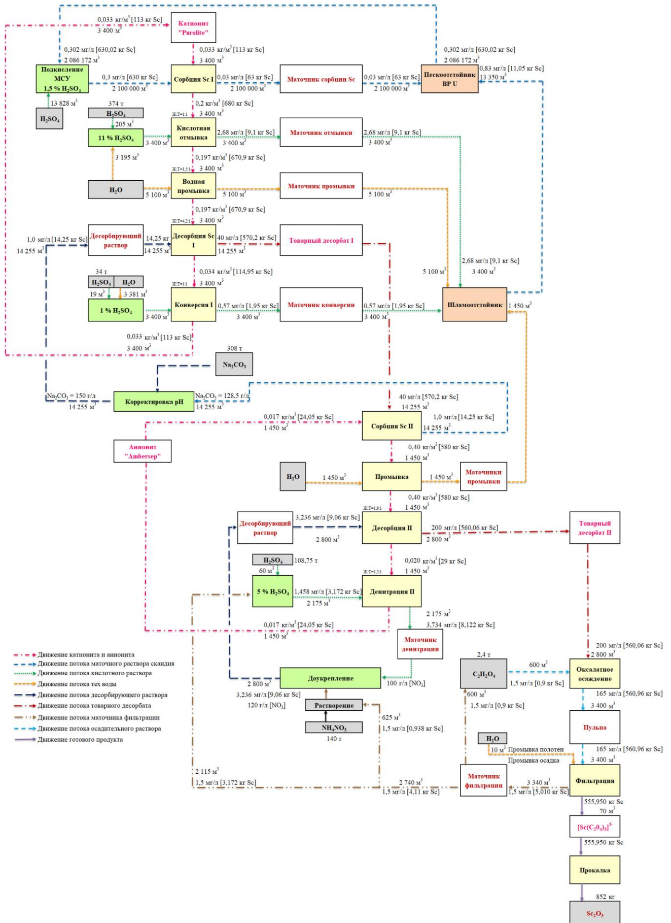
Рисунок 57– Технологическая схема извлечения скандия из МСУ
