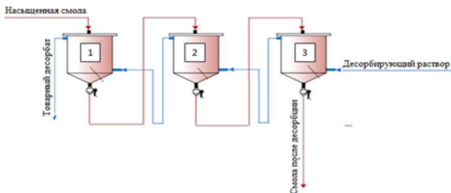
Рисунок 51– Вид каскадной схемы для десорбции скандия с анионита
