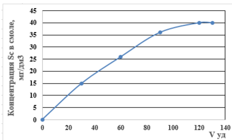
Рисунок 44 – Выходная кривая сорбции Sc ионитом Ambersep 920U, V_{\text{уд}} – отношение объема пропущенного раствора к объему ионита
