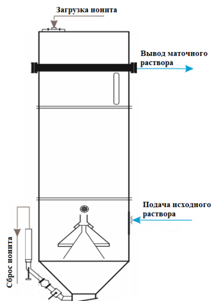
Рисунок 48 – Устройство КИ-1 600
