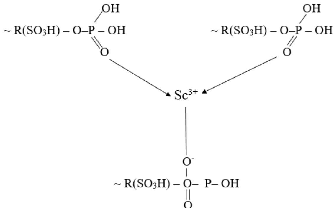
Рисунок 37—Предполагаемая структура ионно- координационного соединения Sc.
