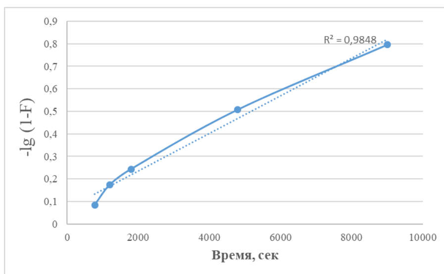
Рисунок 41 – Зависимость -\log(1-F) от времени контакта фаз при сорбции скандия из МСУ на катионите Purolite MTS9580 (Ж:Т= 500, C_{Sc}=0,3 мг/л)
