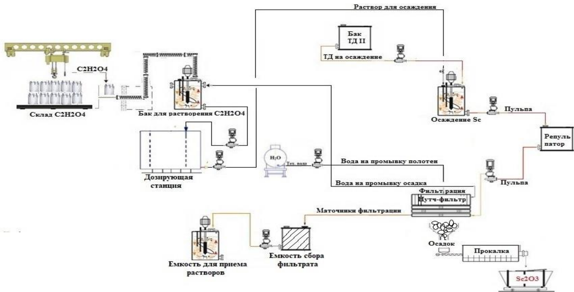
Рисунок 56 – Принципиальная аппаратная схема технологии извлечения скандия (III этап концентрирования) из маточников сорбции урана
