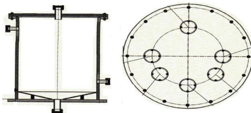
Рисунок 50 – Реактор для десорбции скандия
