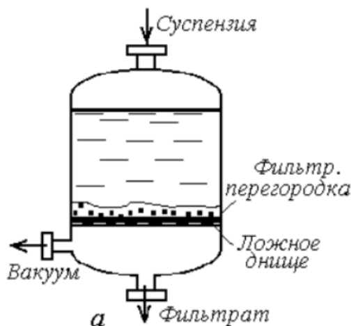
Рисунок 53 – Нутч-фильтр
