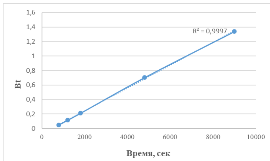
Рисунок 40–Зависимость критерия модели Бойда–Адамса от времени для сорбции Sc из МСУ на катионите Purolite MTS9580 ( H_2SO_4=15 г/дм 3 , Ж:Т= 500, C_{Sc}=0,3 мг/л)
