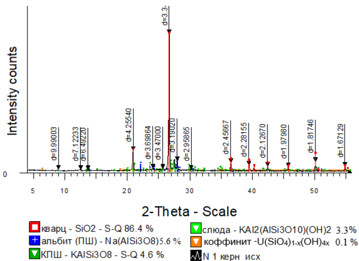
Рисунок 17 – Рентгенофазовый анализ керового материала урановой руды
