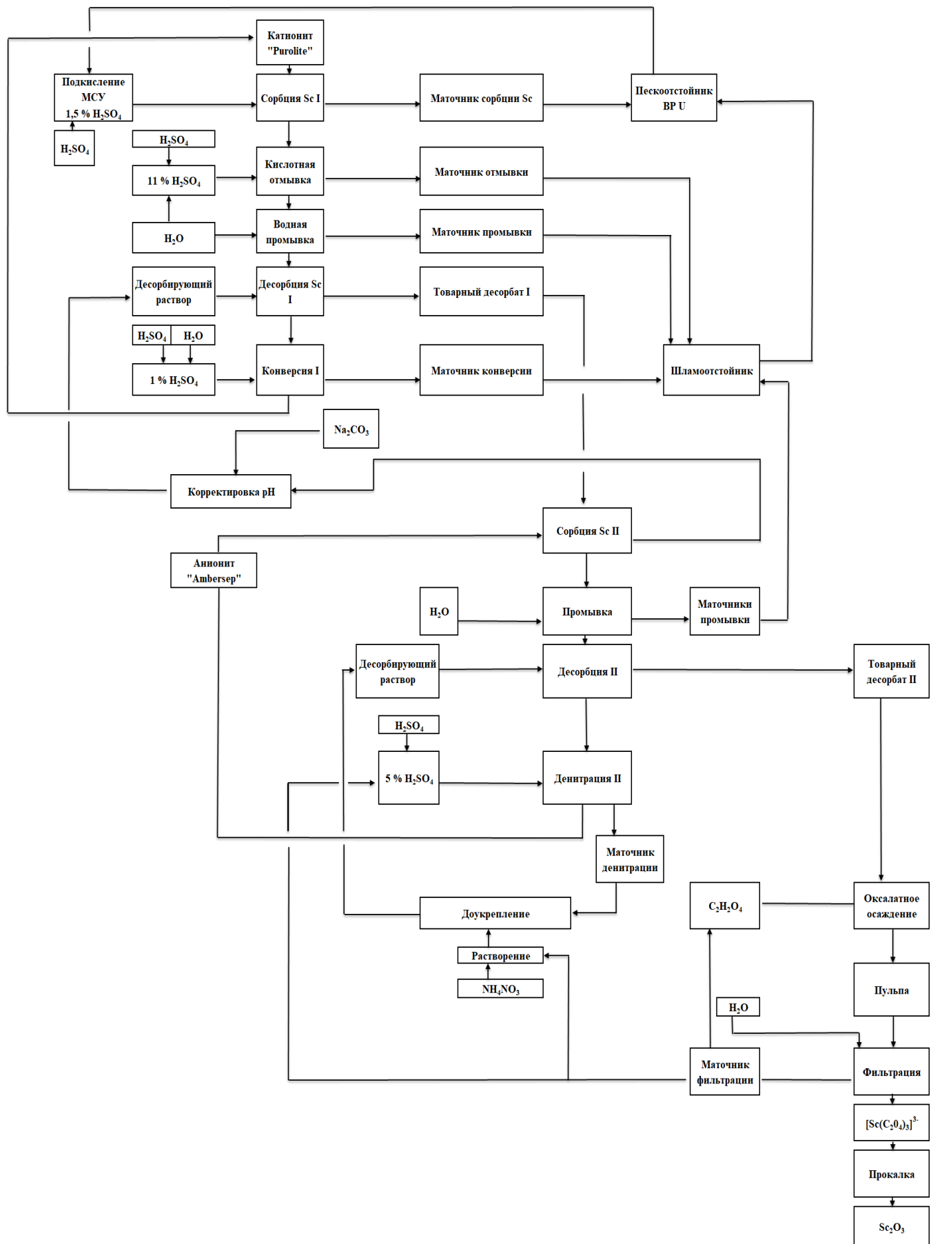
Рисунок 47 – Технологическая схема производства скандия из МСУ
