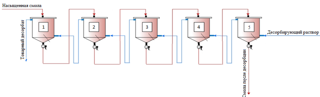
Рисунок 49– Вид каскадной схемы для десорбции скандия
