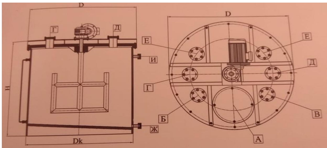
Рисунок 52 – Реактор для осаждения скандия
